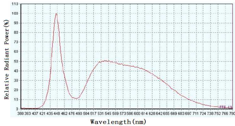
正白光谱图
