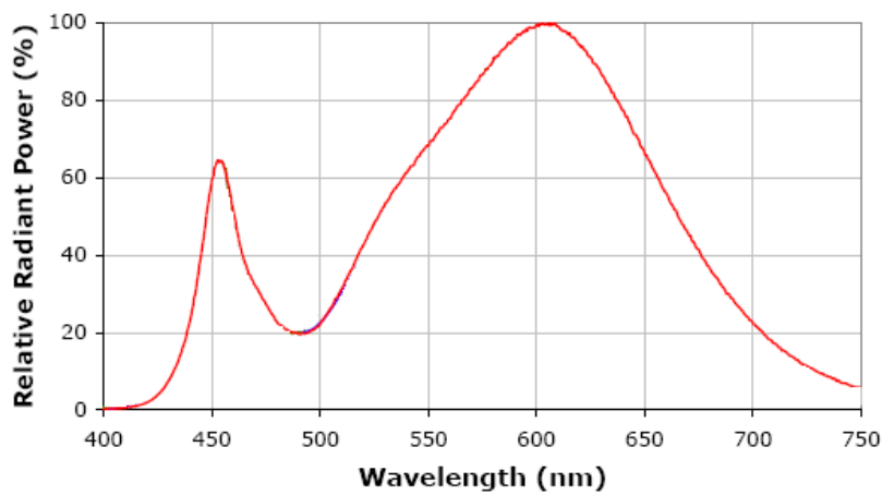
暖白光谱图
